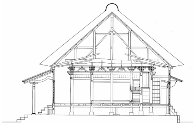
三仏堂修理前断面図
