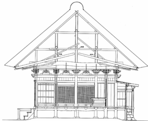
三仏堂現状断面図
